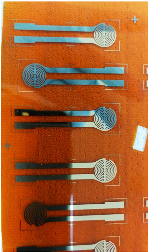
Electrodos desarrollados en la investigación de Zamora.
